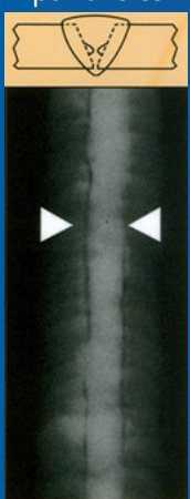
Lignes d'inclision parallèles
