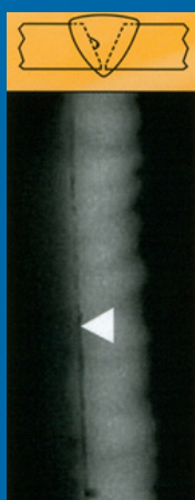
Manque de fusion
