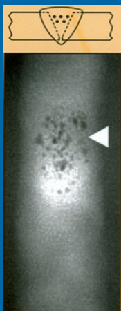
Porosité en grappe
