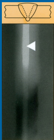
Excès de pénétration
